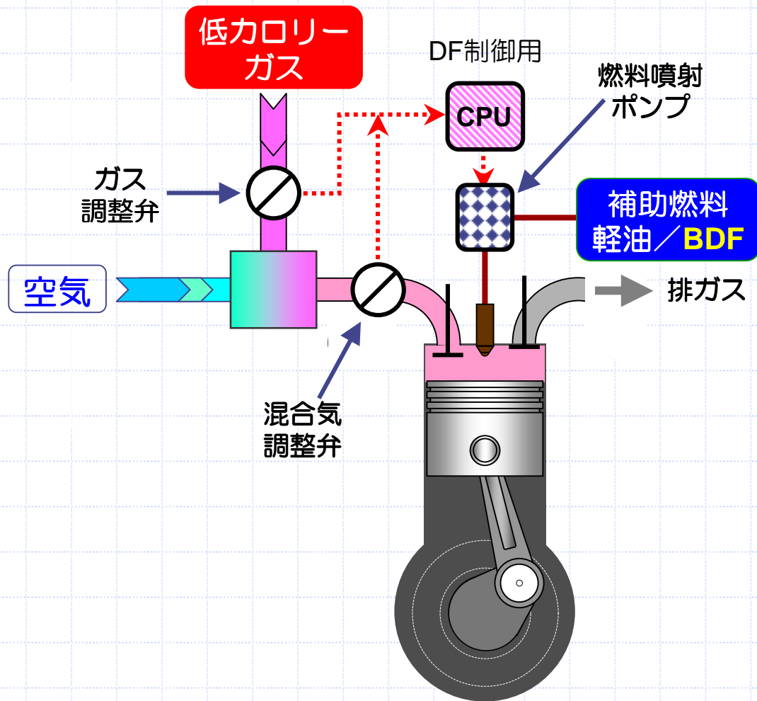
写真1 9.8kW DFコージェネシステム
